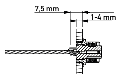
Gewinde-Löcher / Thread holes
