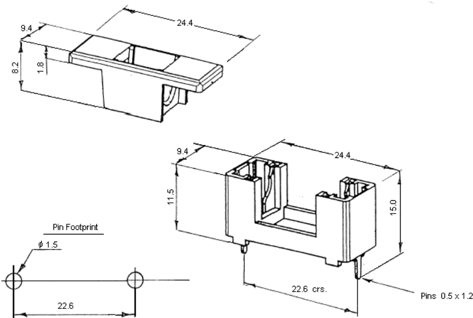
Dimensions : Millimetres
