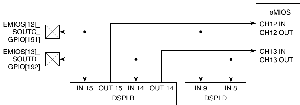
Figure 2-9. EMIO[12:13]—DSPI B—DSPI D I/O Connections
