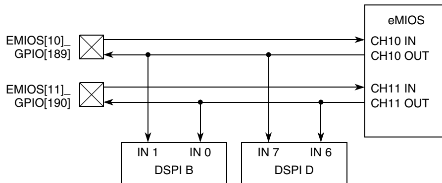
Figure 2-8. EMIO[10:11]—DSPI B—DSPI D I/O Connections
