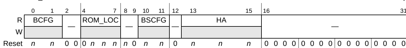
Figure 22-2. POR Boot Mode Status Register (PORBMSR)
