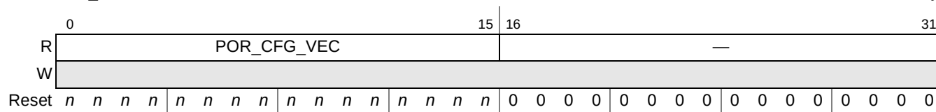
Figure 22-6. POR Configuration Register (GPPORCR)
