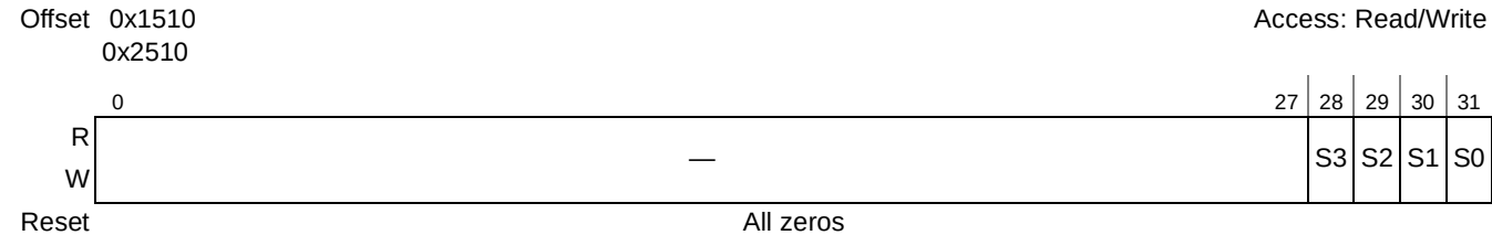
Figure 9-30. Message Status Register (MSR)
