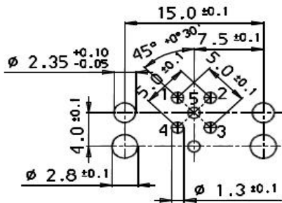
Leiterplattenbohrbild K-Seite
