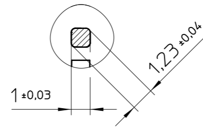
Teilansicht1 5:1
