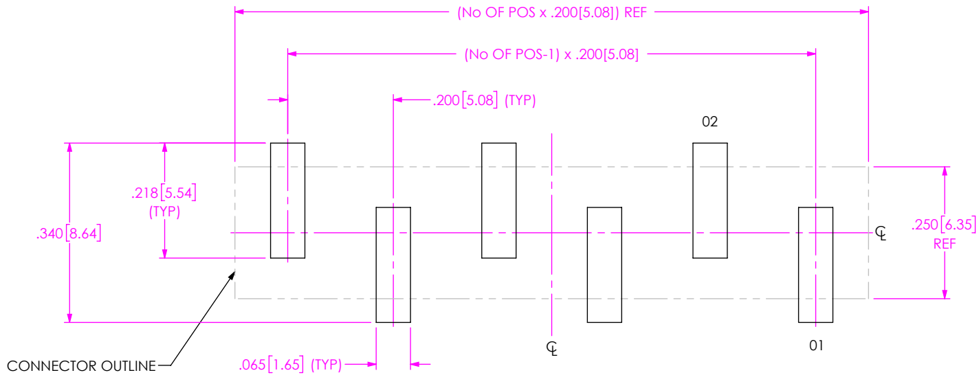
FIG 2 HPM-XX-XX-XX-S-VS-X SHOWN (FOR -S-VS OPTION)
