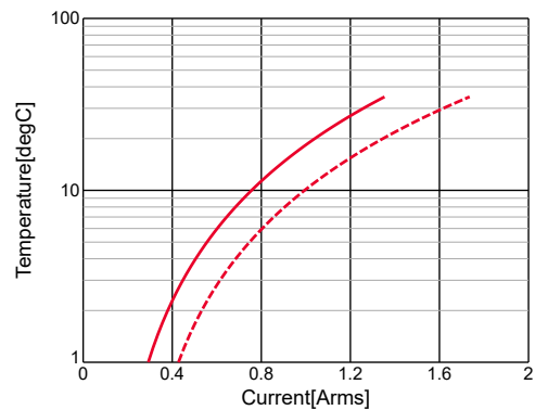
GRM155R60J154KE01#,Temp.rise 500kHz 1MHz
