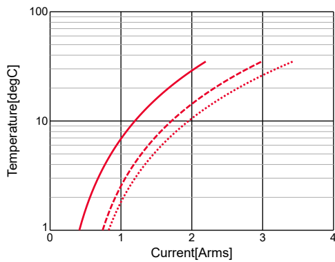
GRM155R60J824KE19#,Temp.rise
