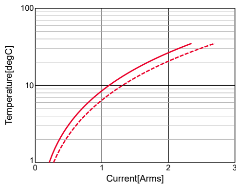
GRM185R60J105KE26#,Temp.rise
