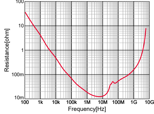
GRM188R71E224KA88#,R,DC0V,25degC
