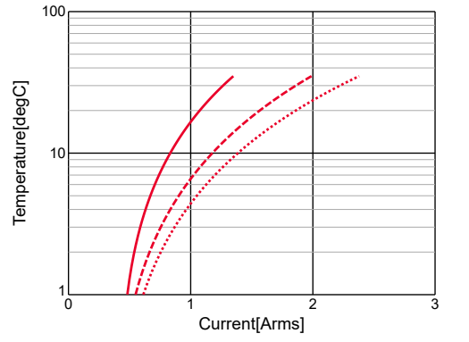
GRM188R71E224KA88#,Temp.rise
