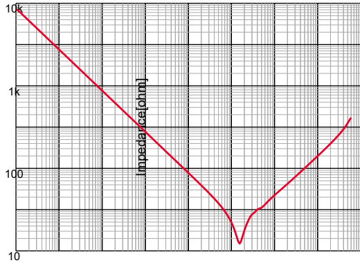
GRM188R71E224KA88#,|Z|,DC0V,25degC
