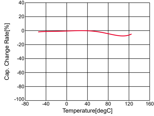
C-Temp.(Cap Change)
