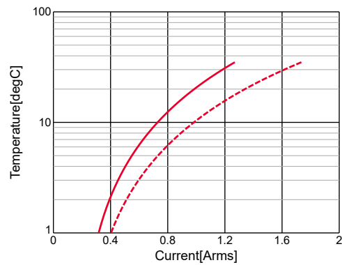
GRM188R71H104KA93#,Temp.rise
