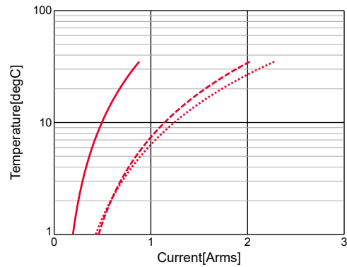
GRM21BR71C224KA01#,Temp.rise
