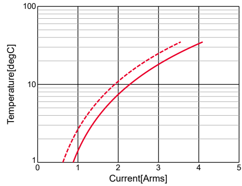
GRM21BR71H105KA12#,Temp.rise 500kHz 1MHz
