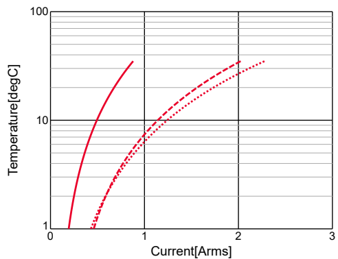
GRM21BR71H224KA01#,Temp.rise
