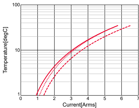
Temp.rise
