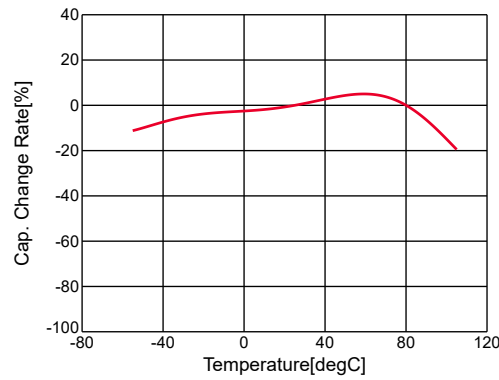
C-Temp.(Cap Change)
